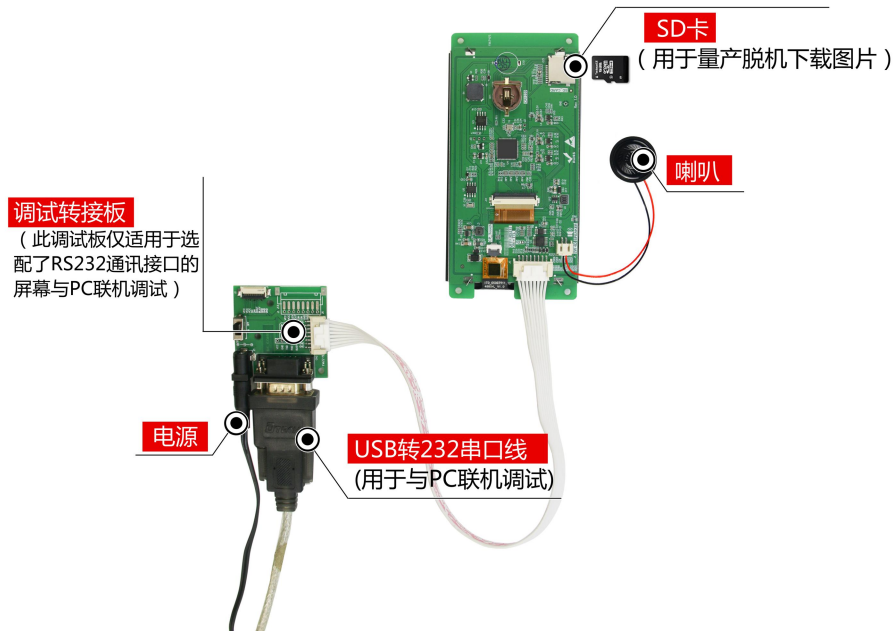
图 1-4 调试工具图
