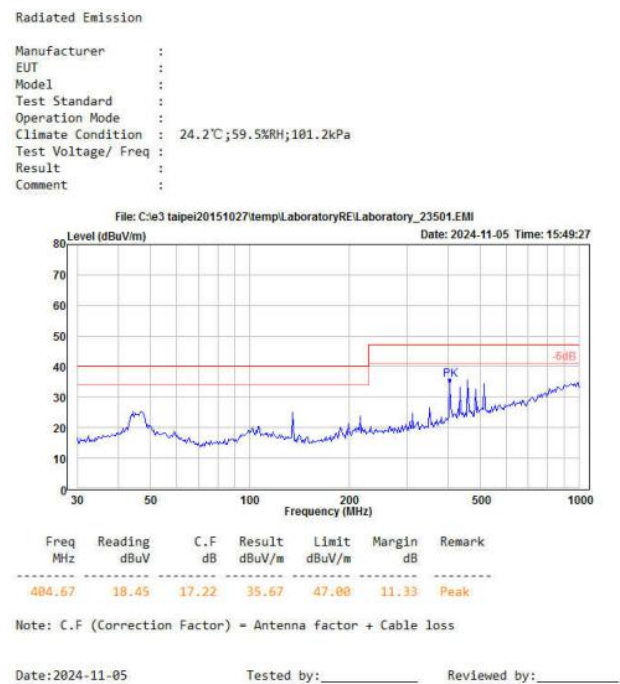
图 4-6 RE 测试垂直方向
