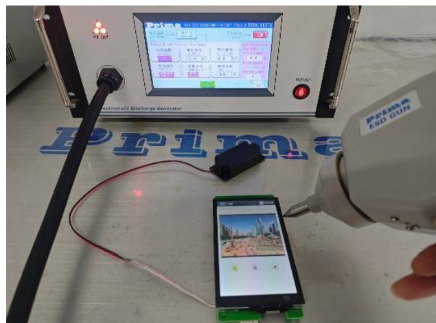
图 4-2 ESD 测试图
