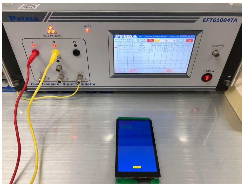
图 4-3 EFT 测试图
