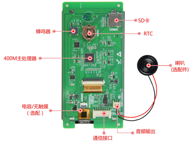
图 1-3 硬件配置图
