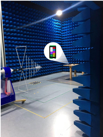
图 4-4 RE 测试图
